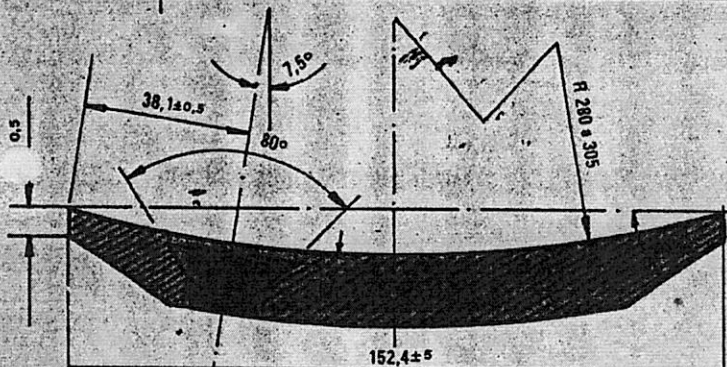
SECCION A - B SECTION A - B
